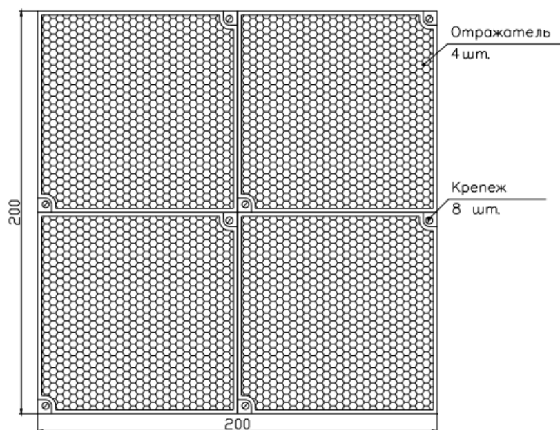
Рисунок 2 - Общий вид пластины со смонтированными на ней четырьмя отражателями
