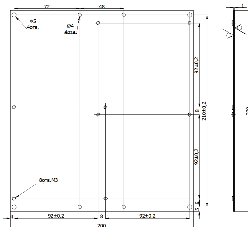
Рисунок 1 - Общий вид пластины для установки четырех отражателей
